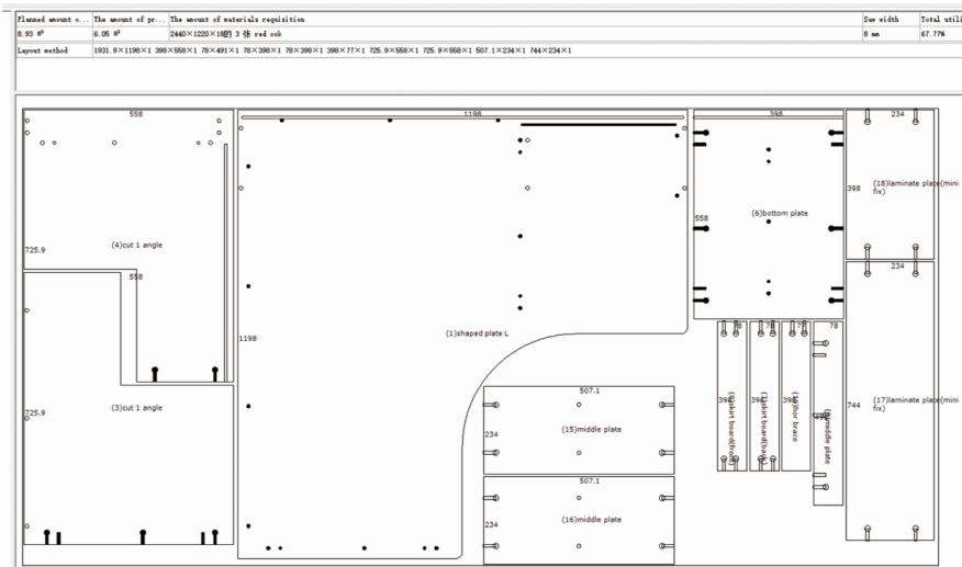
Sơ đồ tối ưu ván
